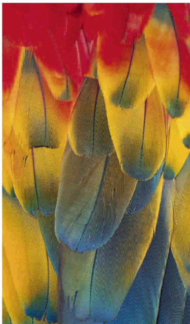
Οι επικαλυπτόμενες δομές των φτερών τα καθιστούν ελαφρά αλλά ανθεκτικά. Στο λεύκιμμα «Νανόκοσμος» (εκδ. Καπόν).
